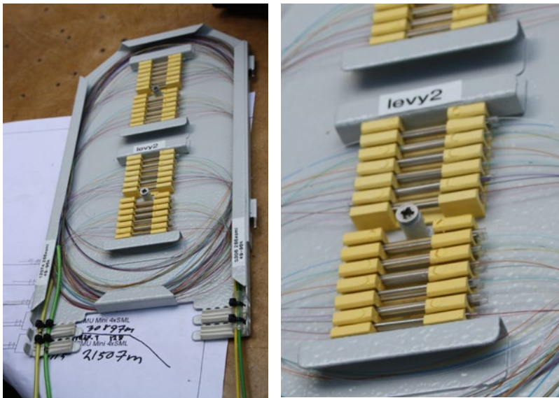
Kuva 8.5. Kuitujatkossuojia jatkoslevyllä (Kuvat: Nestor Cables Oy).
