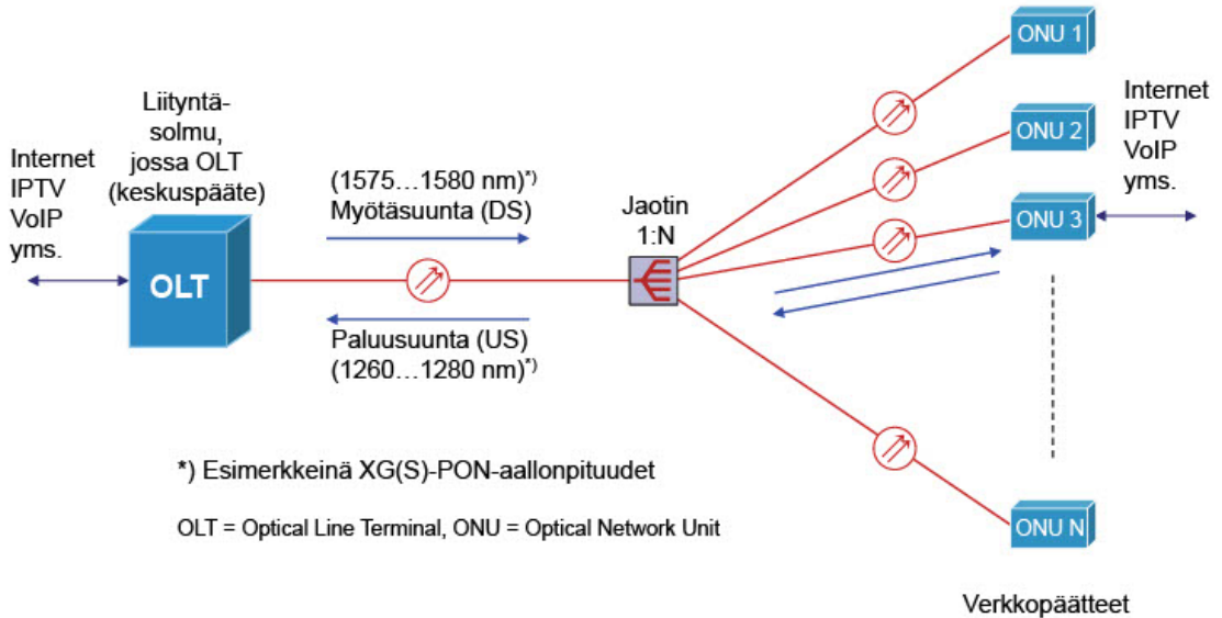
Kuva 5.12. PON-verkon periaate.
