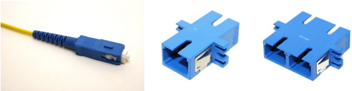
Kuva 4.5. SC-liitin ja SC-adaptteri.
