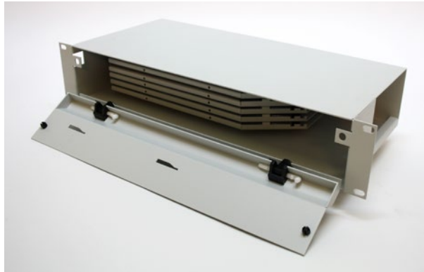
Kuva 4.31. 19 tuuman telineeseen tai kaappiin asennettava sisäjatkoskotelo (Nestor Cables Oy).
