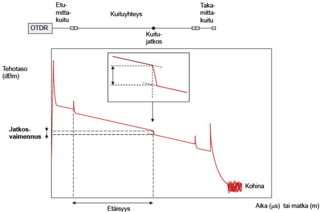
Kuva 9.11. Jatkosvaimennuksen mittaamisen periaate.
