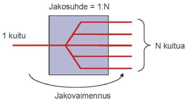
Kuva 4.15. Jaottimen periaate sekä yleisimmät jakosuhteet ja niitä vastaavat tyypilliset jakovaimennukset.
