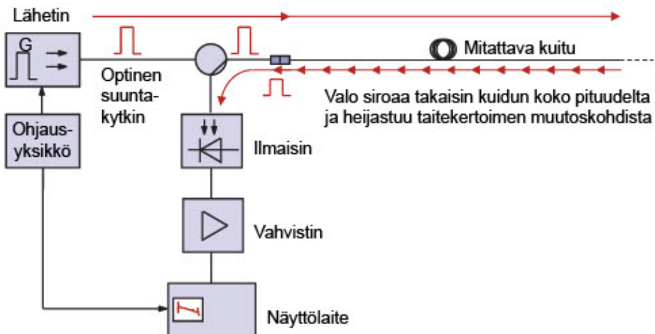
Kuva 9.6. Valokaapelitutkan toimintaperiaate.
