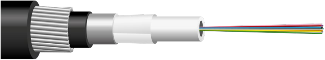
Kuva 3.8. Pyörölanka-armeerattu vesistökaapeli.
