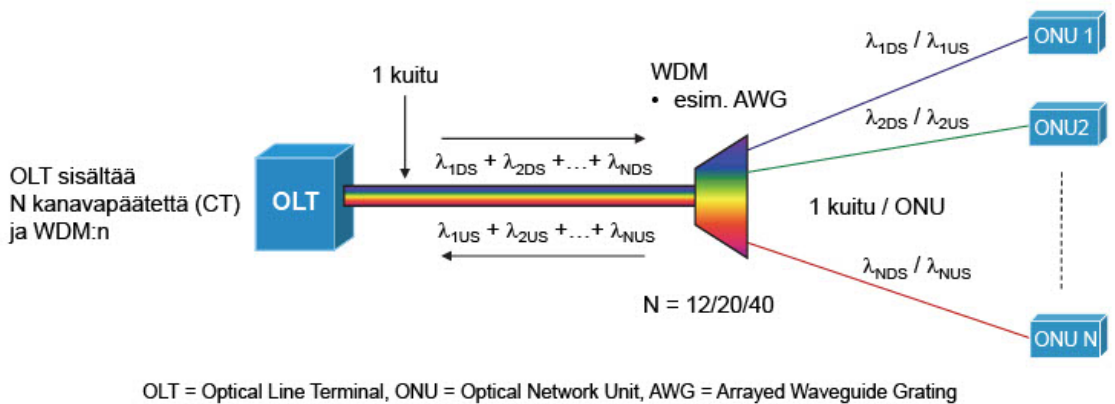
Kuva 5.20. WDM-PON-verkon periaate.
