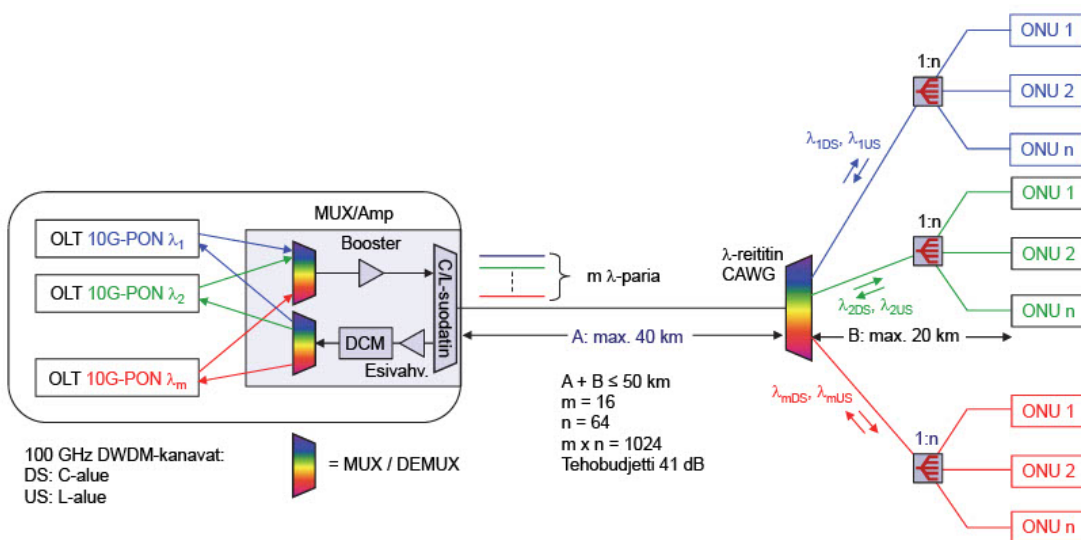
Kuva 15.21. Super-PON.
