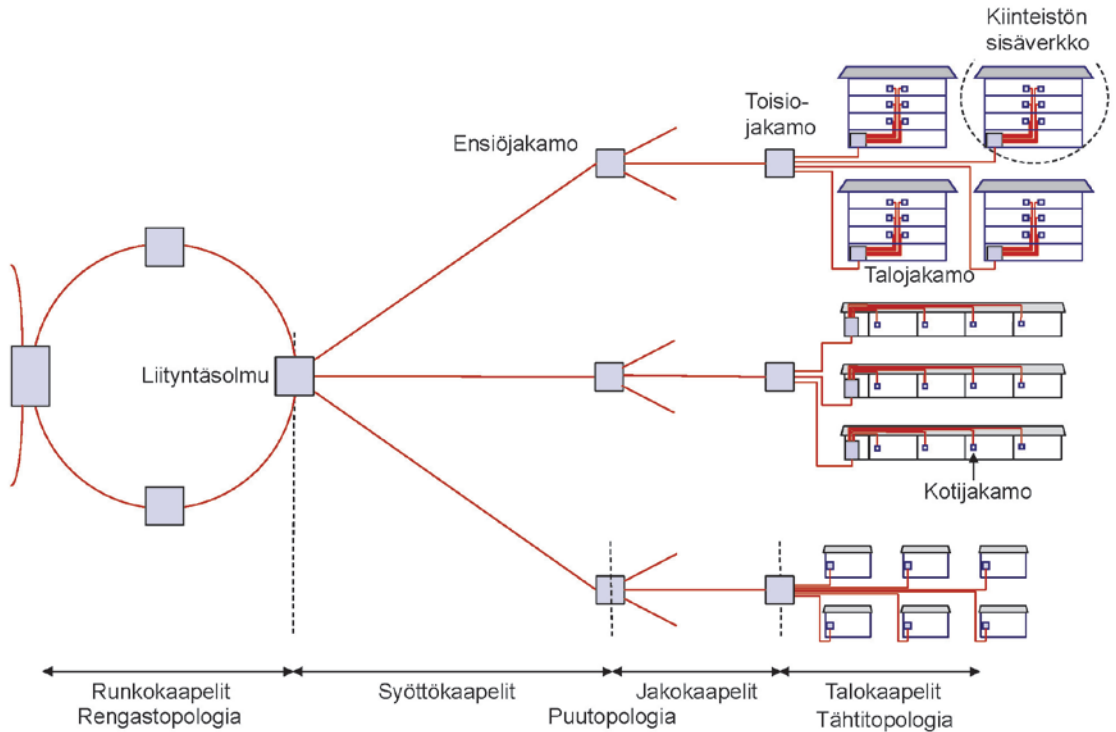
Kuva 6.4. Optisen liityntäverkon perusmalli (referenssimalli).
