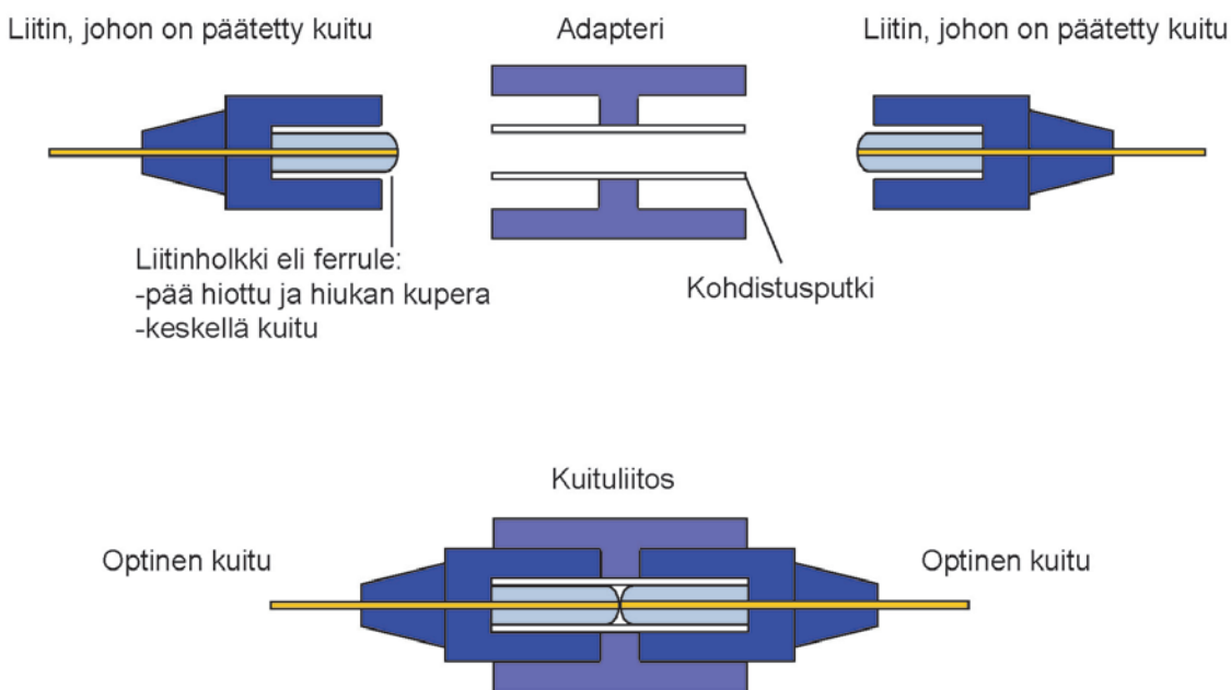
Kuva 4.2. Holkkiliittimen perusrakenne.
