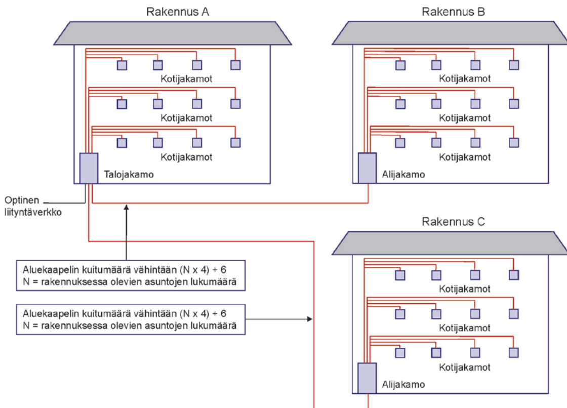
6.21. Samaan kiinteistöön kuuluvien asuinkeuhkotalojen välinen optinen kaapelointi.
