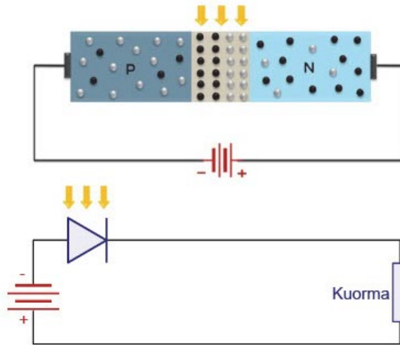
Kuva 5.25. Valodiodin toimintaperiaate.
