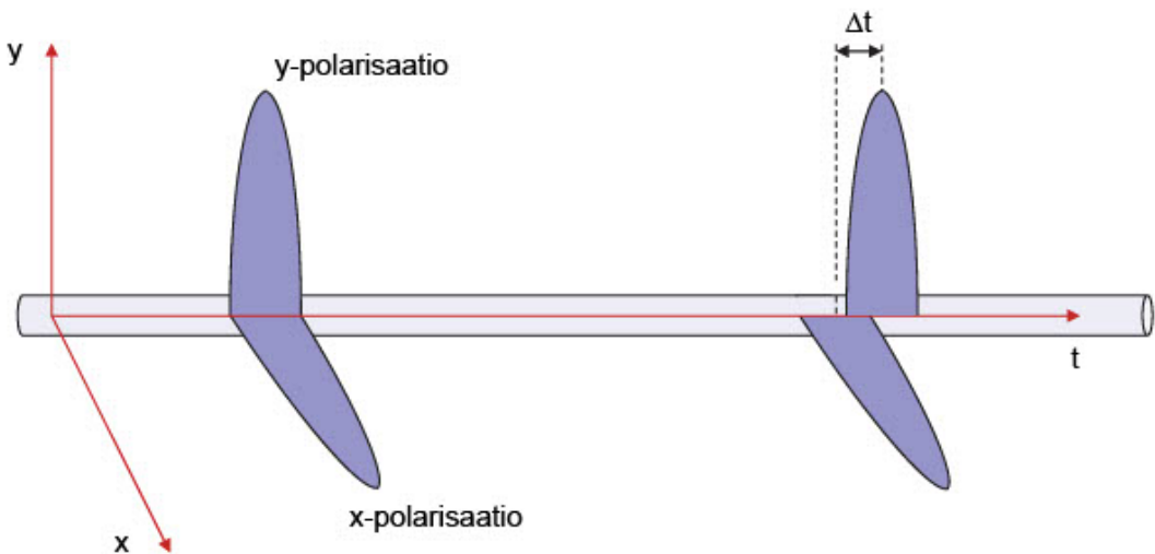
Kuva 2.13. Eri polarisaatiomuodoissa (x- ja y-polarisaatio) etenevillä valonsäteiden komponenteilla on hiukan erisuuruiset nopeudet. Tämä aiheuttaa kulkuaikaeroa, jota kutsutaan polarisaatiomuotodispersioksi.
