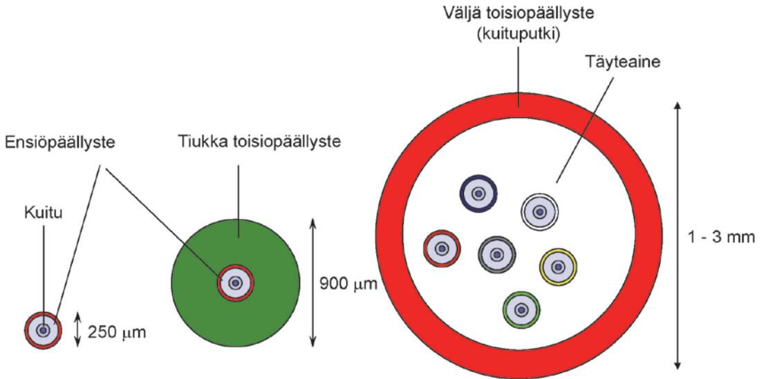
Kuva 3.1. Ensiöpäälyste, tiukka toisiopäälyste ja väljä toisiopäälyste.
