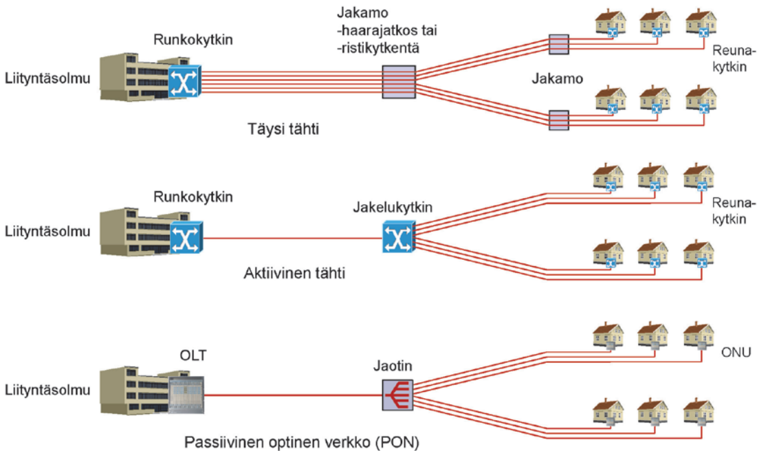
Kuva 6.2. Kolme kuitutopologiaa.
