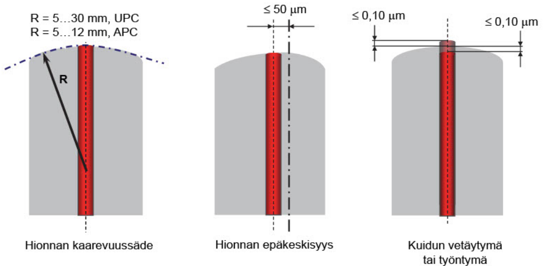
Kuva 4.4. Hionnan tunnusluvut.
