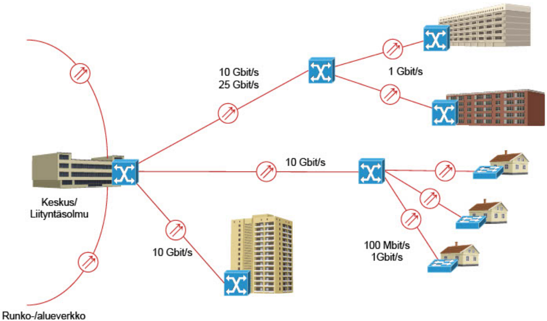
Kuva 5.9. Point-to-point-topologian mukainen optinen Ethernet-liittytverkko.
