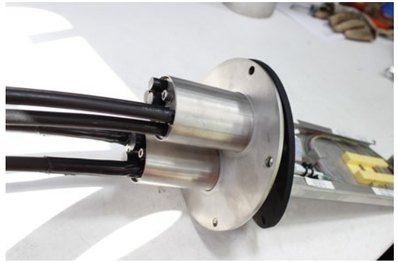
Kuva 4.28. Asennettuja ulkojatkoskoteloita (Kuvat Nestor Cables Oy).
