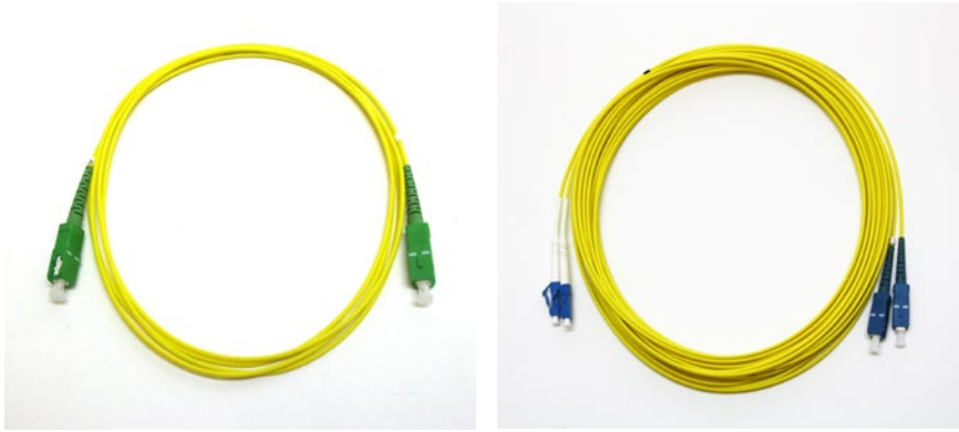
Kuva 4.14. Esimerkkejä kytkentäkaapeleista.
