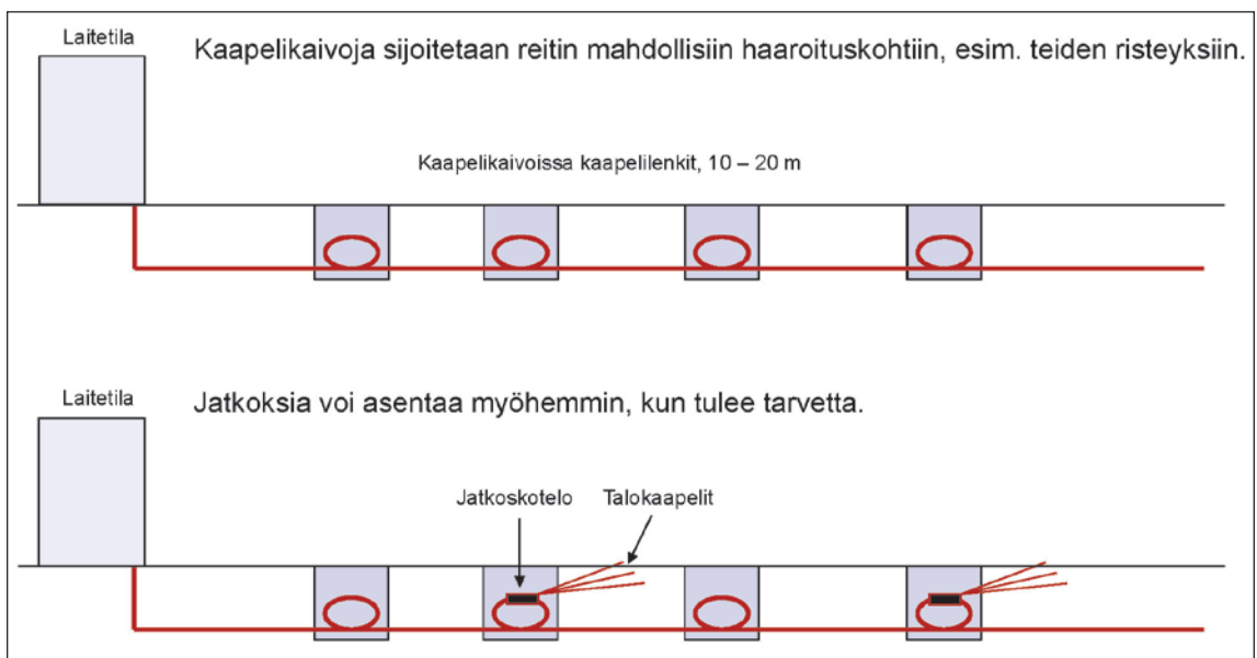
Kuva 8.11. Kylkioton hyödyntäminen maaseutualueella.
