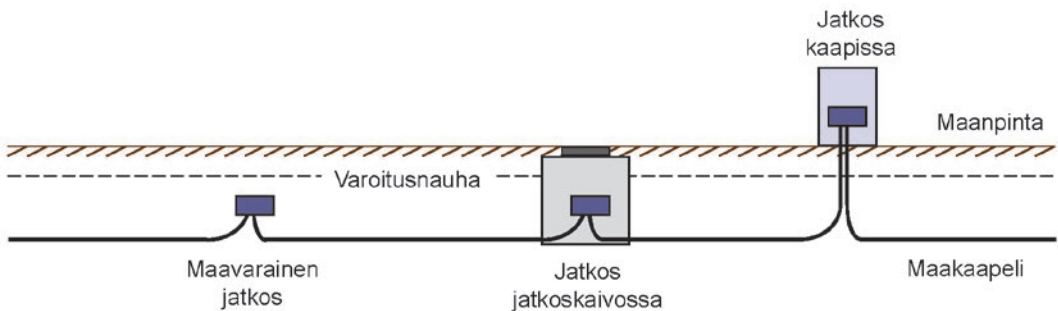
Kuva 7.18. Maakaapelijatkos voidaan sijoittaa suoraan maahan, jatkoskaivon tai kaappiin.
