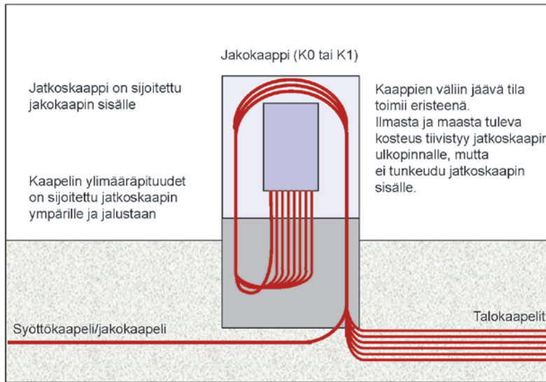
Kuva 8.9. Jatkoskaapin periaate.
