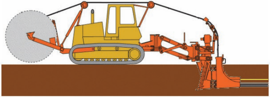
Kuva 7.16. Kaapelin auruksen periaate. (Kuva: Lancier Cable GmbH).
