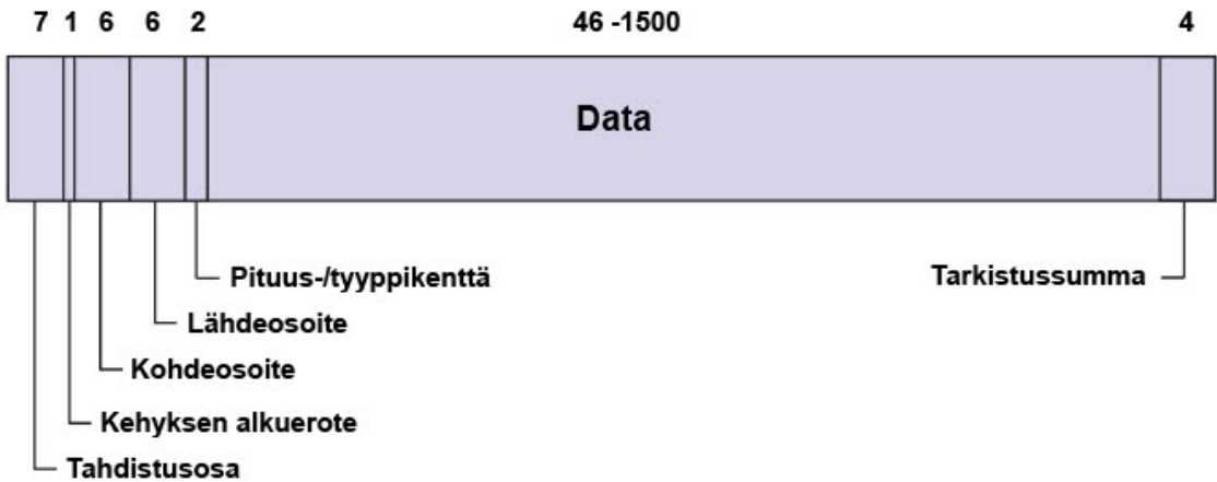
Kuva 5.10. Standardin IEEE 802.3 mukaisen Ethernet-kehuksen rakenne.
